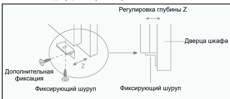
Рис 14: Регулировка нижнего торца дверцы шкафа
