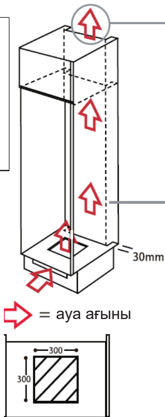
Желдету саңылауларын кесу схемасы
